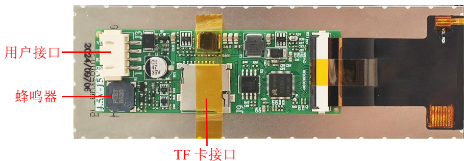
图 1 产品外观及硬件配置图
