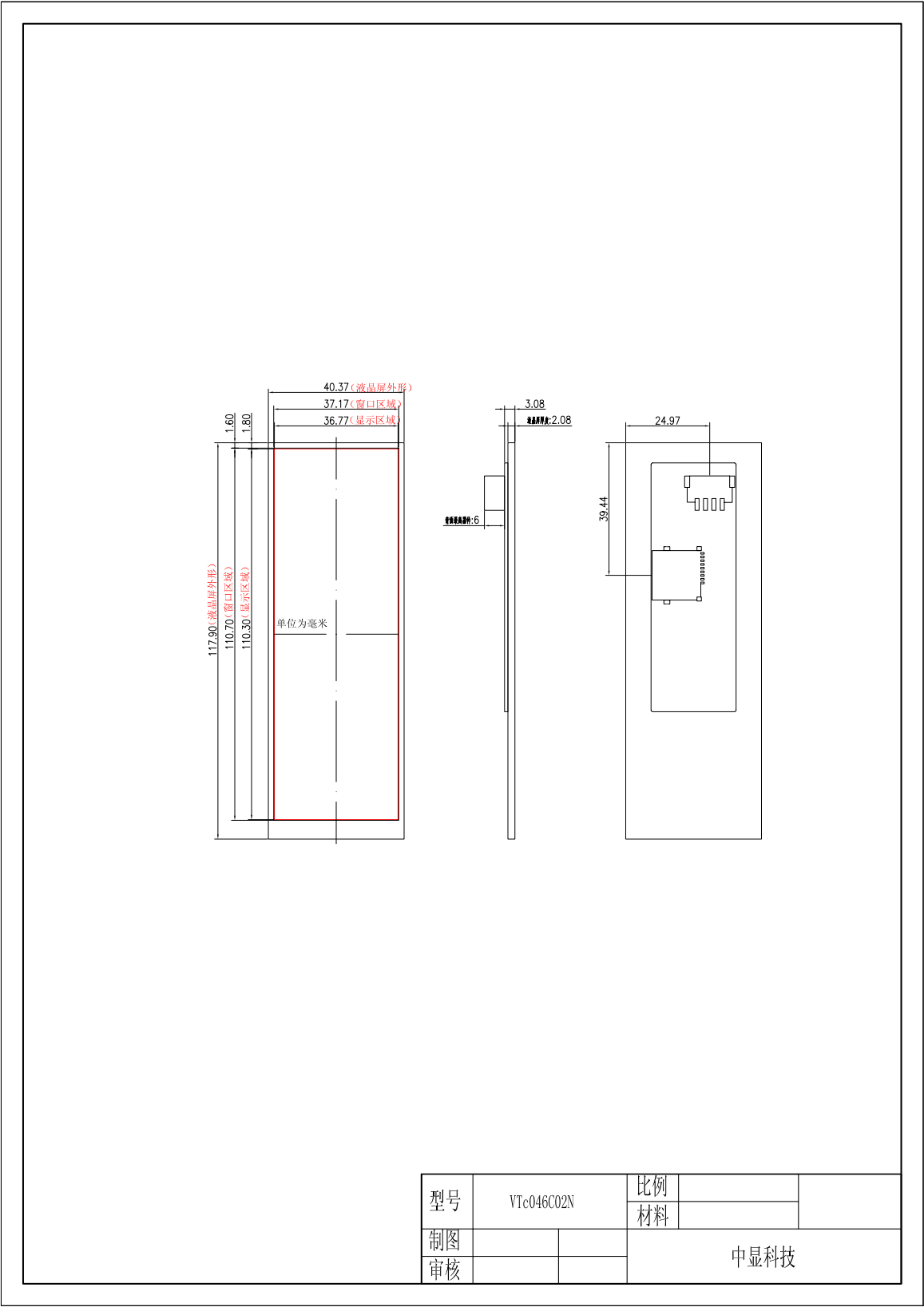
图 2 VTc046C02N 尺寸图
