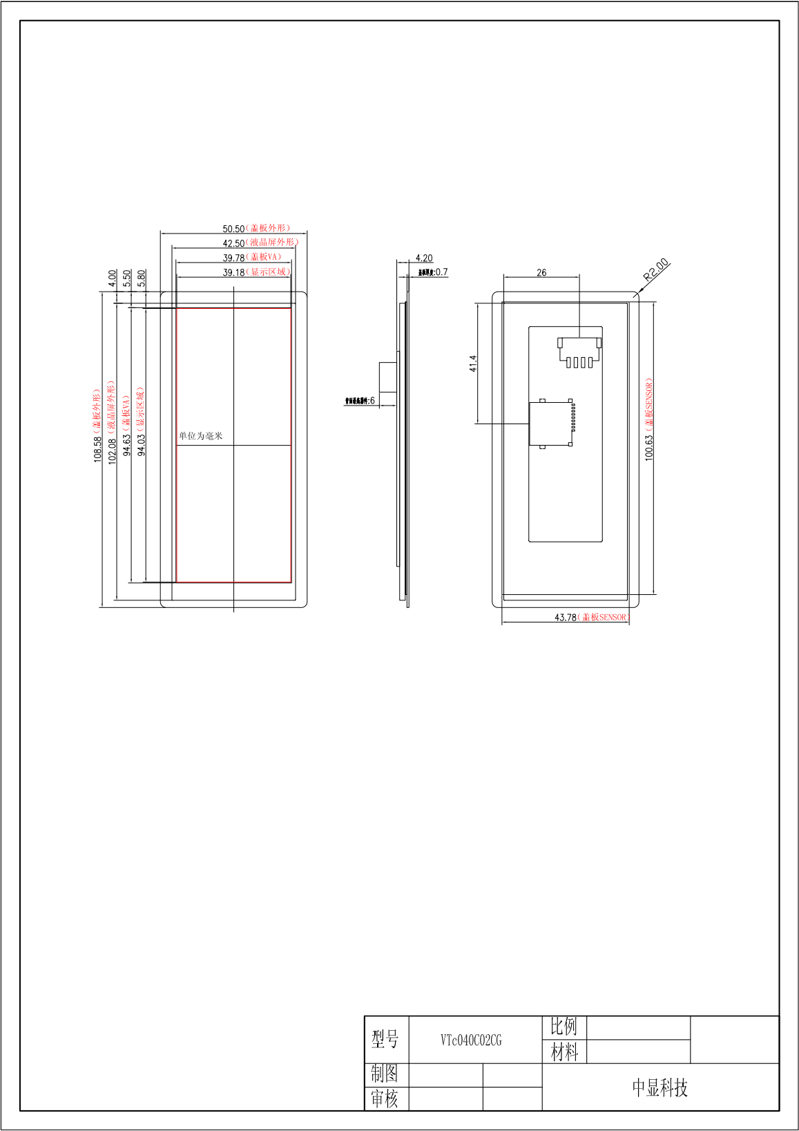
图 3 VTc040C02CG 尺寸图
