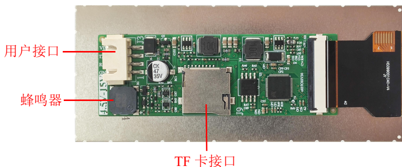
图 1 产品外观及硬件配置图
